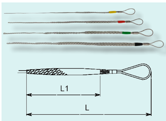
Calza tiracavi di testa per conduttori aerei.
