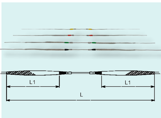
Calza tiracavi di giunzione per conduttori aerei.
